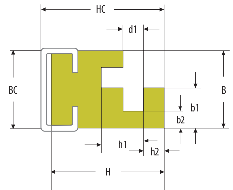
PROFIL - CKRS
