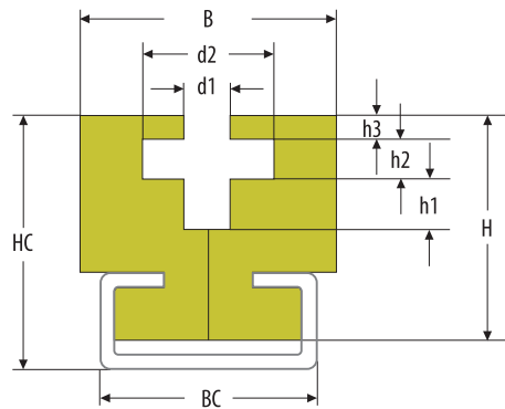
PROFIL - CKR
